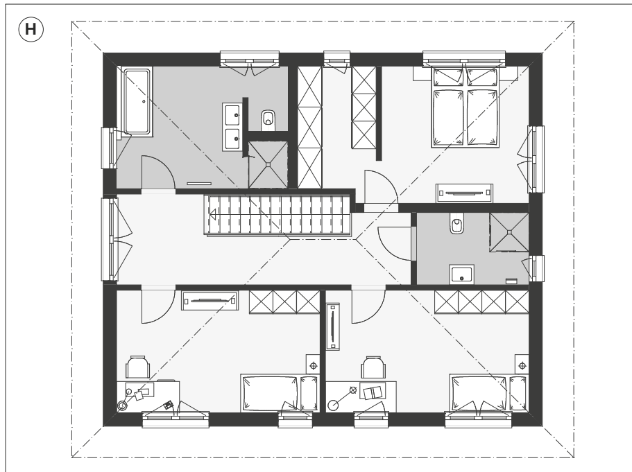
Variante mit 3 Zimmer und DU/WC
