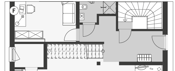
Variante Eingang Osten mit offener Treppe (Musterhaus) + Kellertreppe
