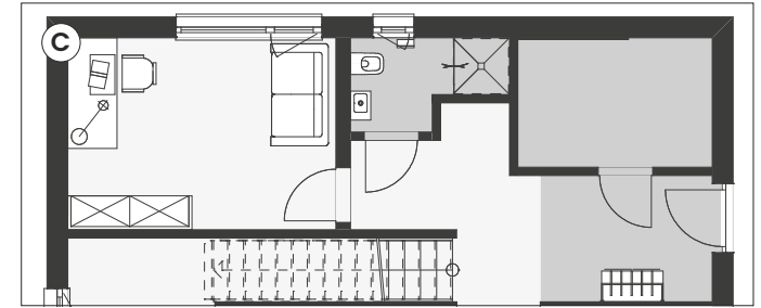
Variante Eingang Osten
