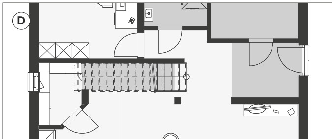
Variante Eingang Osten mit offener Treppe (Musterhaus)
