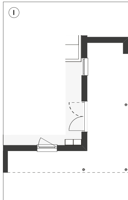
Eck-Terrassenüberdachung Design 130 x 763 / 250 x 814 cm
