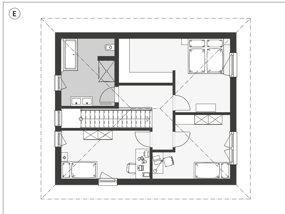
Variante mit großem Bad im OG
