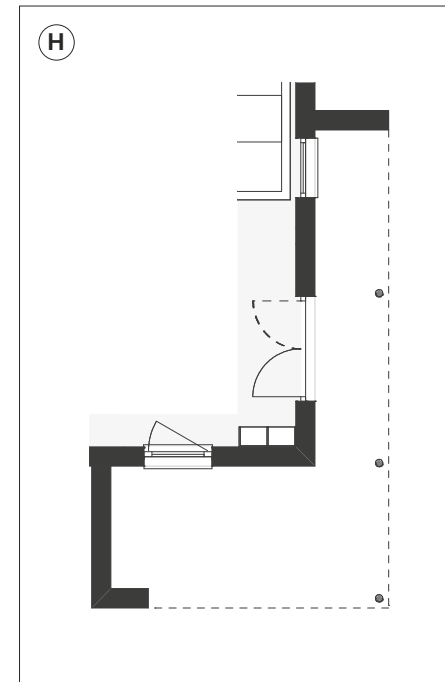
Eck-Terrassenüberdachung Design 130 x 867 / 250 x 524 cm
